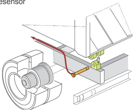
Boltlastcellesensor
